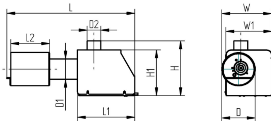
Σχήμα 2 Διαστάσεις
